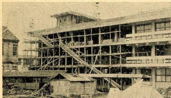
北中学校舎
