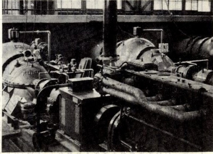
玄好町の下水中断ポンプ場内部
