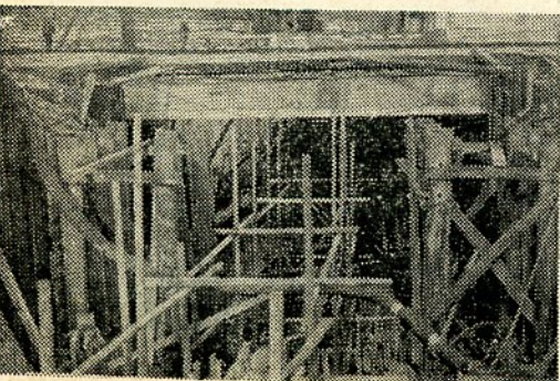
④小南屋裏の鉄道立体交差工事。地下トンネル。地帯と市街を直結する
