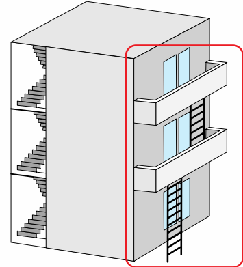
避難上有効なバルコニーの設置
