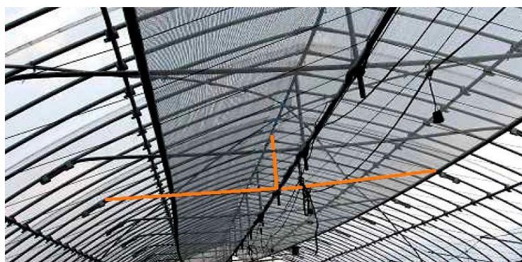
写真1 タイバー設置の例
