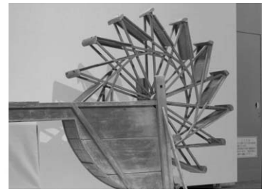
踏み車 ふみぐるま (揚水器)
