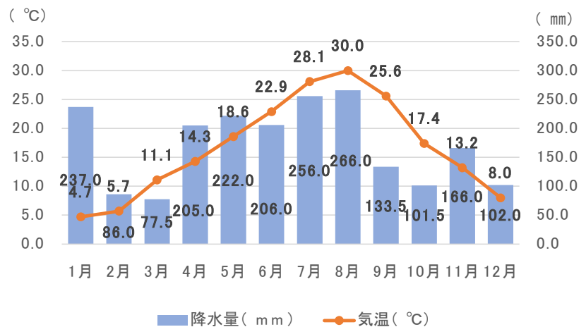
気温、降水量
