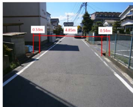
市道大学通り 現況写真①
