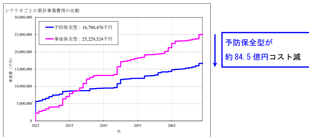
図 5.2 中長期における1,311橋のLCC（前回計画）
