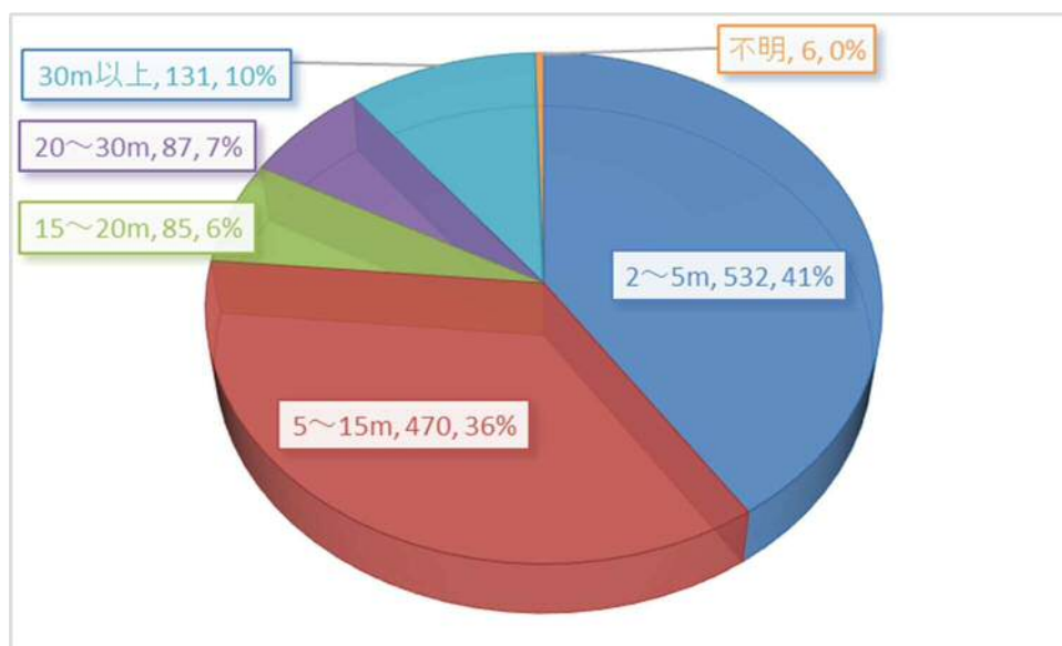
図-2.3 橋長の分類
