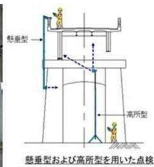
ロボットカメラを使用した点検
