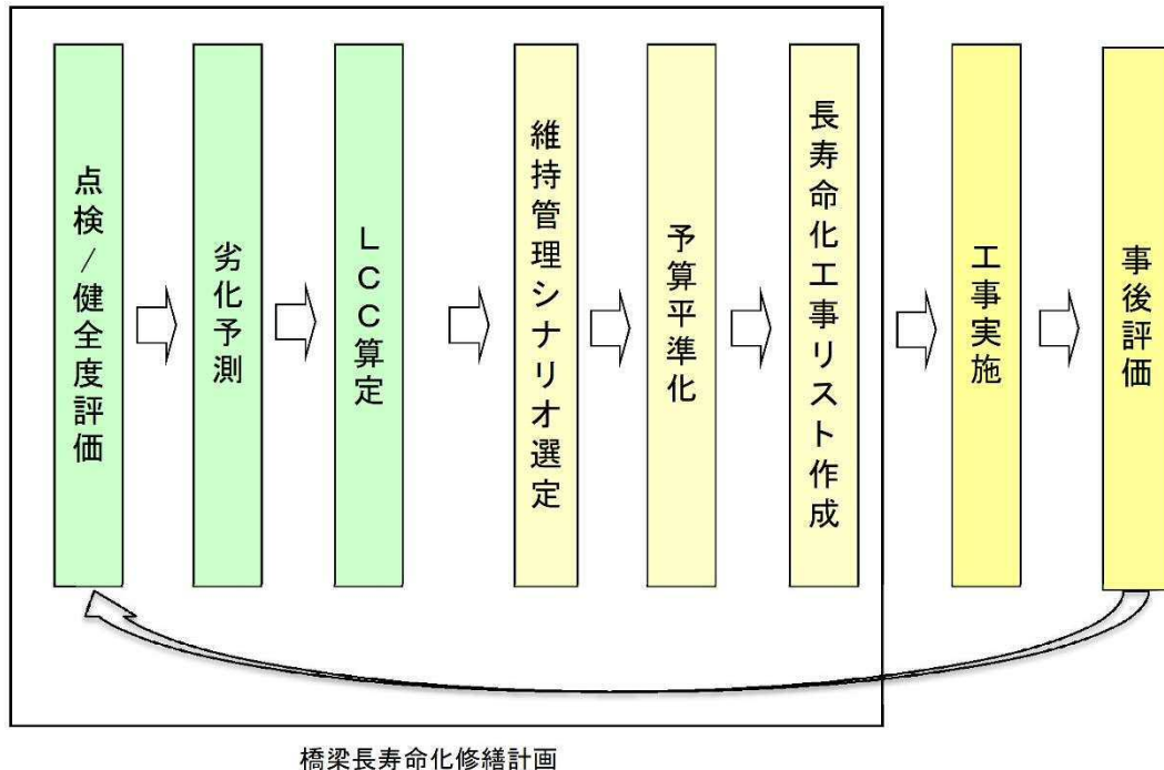
図-4.1 橋梁長寿命化修繕計画のフロー
