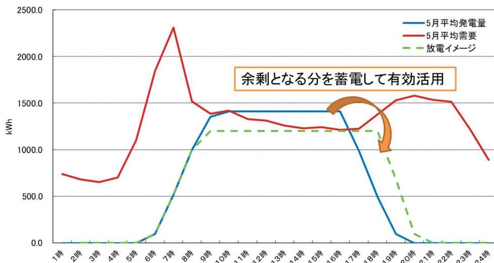
グラフ：若葉台エリア野立てメガソーラー（3.7MW）併設の蓄電池（2MWh）の運用イメージ
