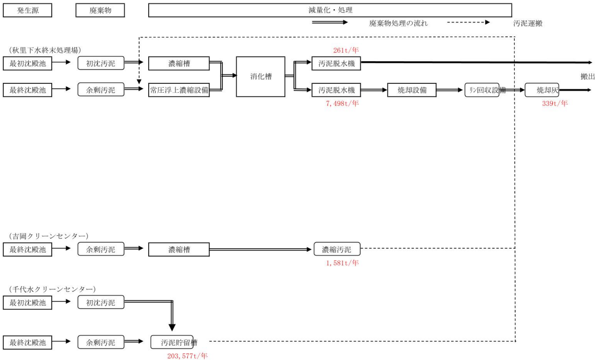
廃棄物処理フローシート
