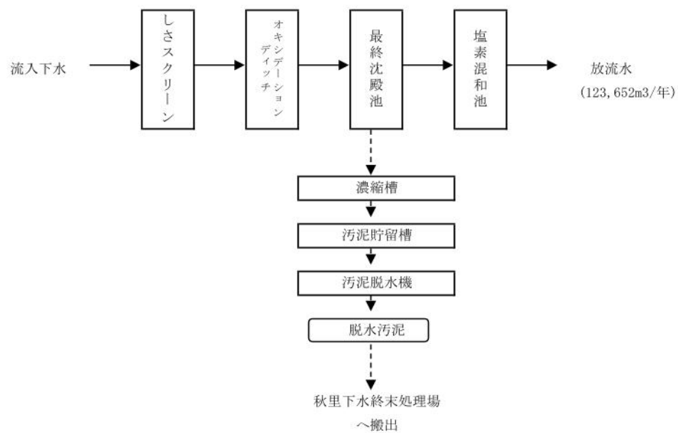
図8 鹿野浄化センター処理フローシート
