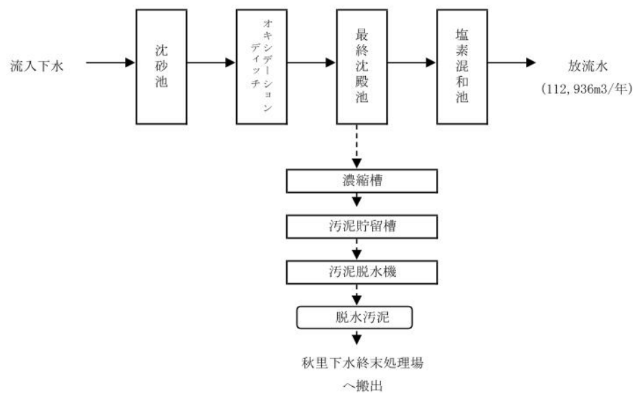
図6 用瀬浄化センター処理フローシート
