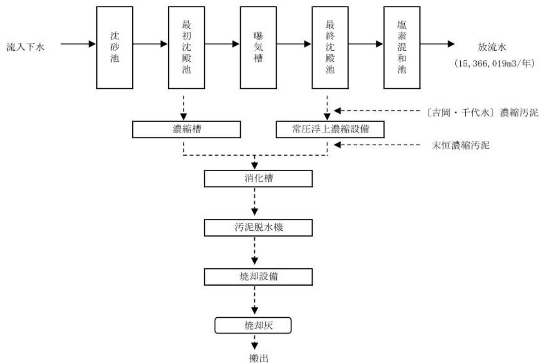
図1 秋里下水終末処理場処理フローシート
