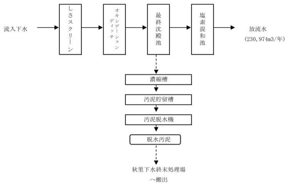
図10 青谷浄化センター処理フローシート
