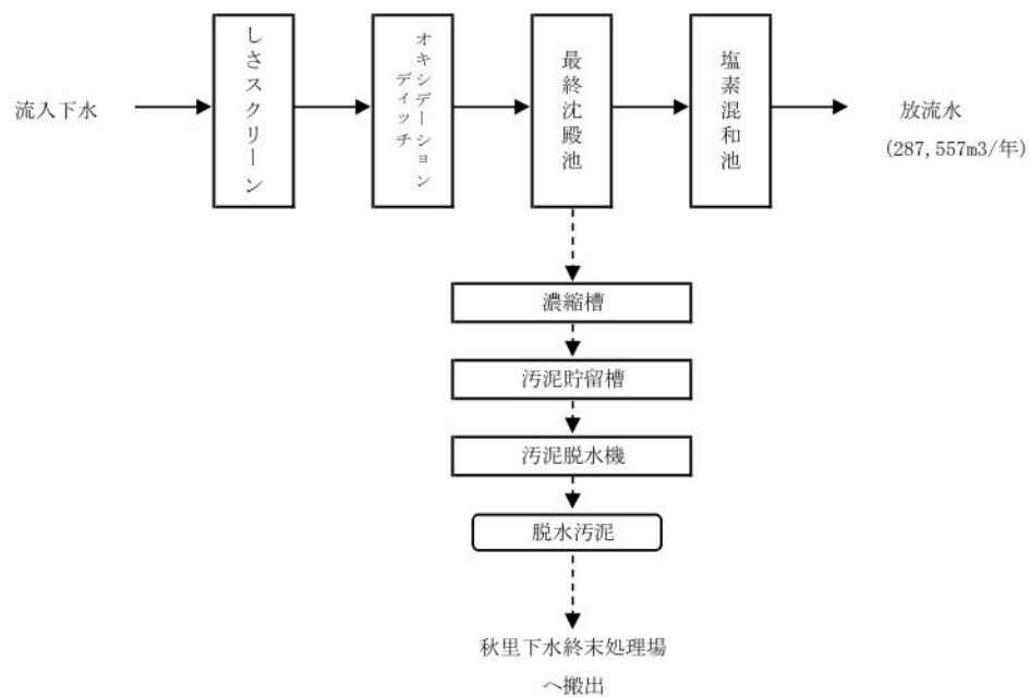
図 10 青谷浄化センター処理フローシート
