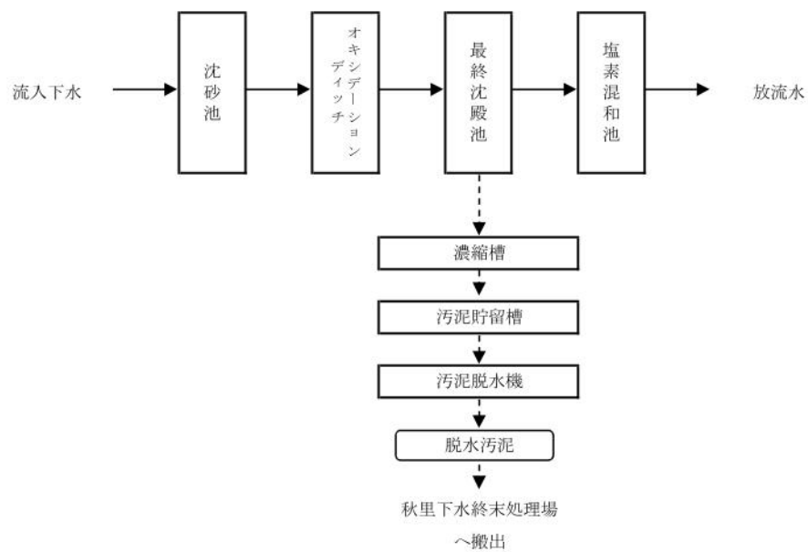
図6 用瀬浄化センター処理フローシート
