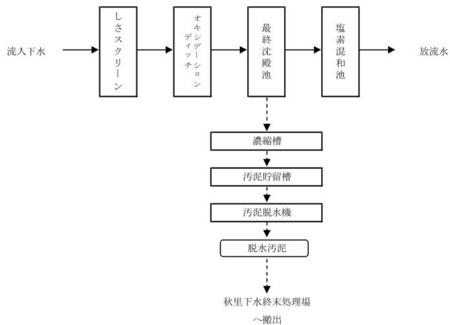
図8 鹿野浄化センター処理フローシート
