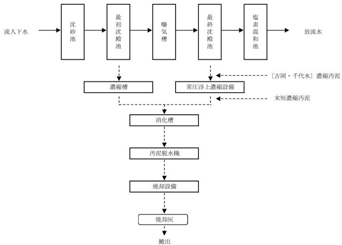
図1 秋里下水終末処理場処理フローシート
