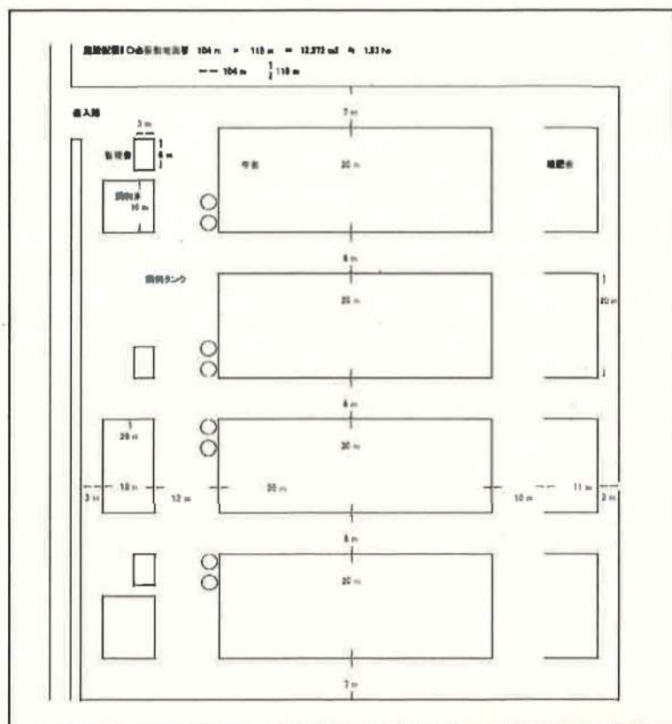
■施設平面図
