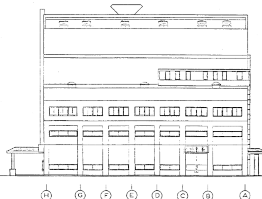
東側立面図 1/200
