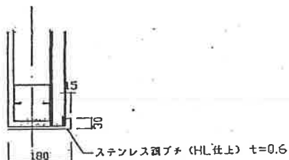
B部水平断面詳細
