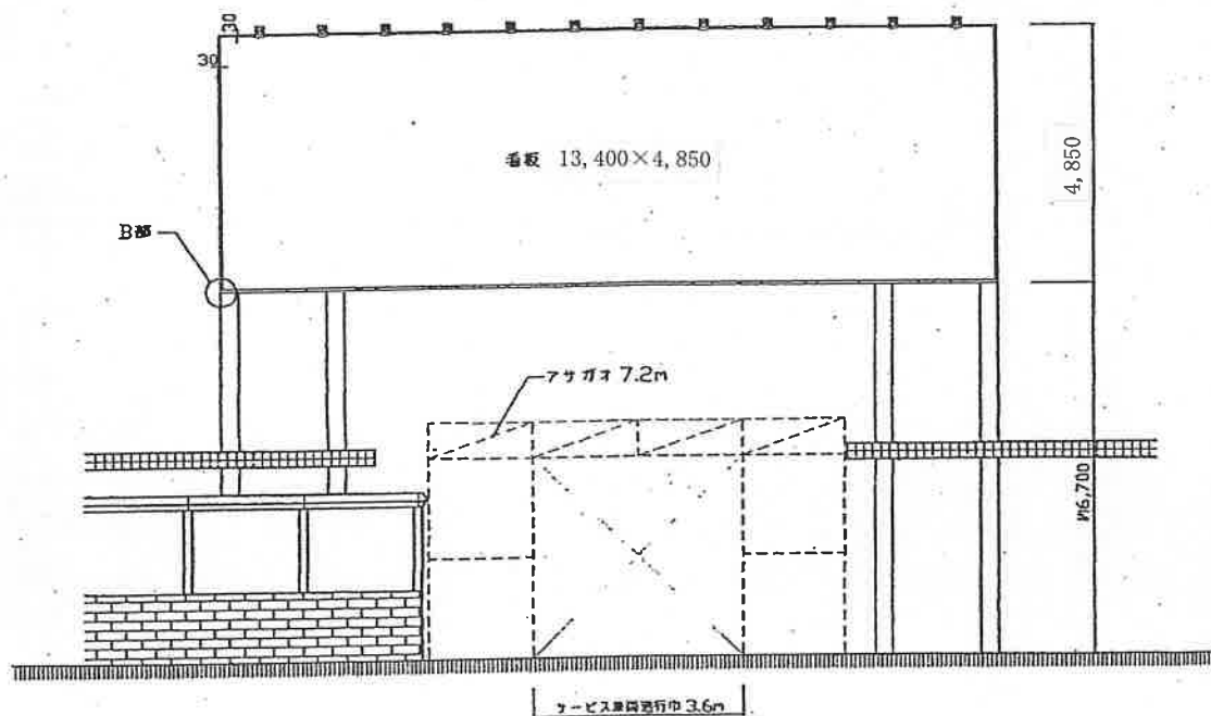
立面図
