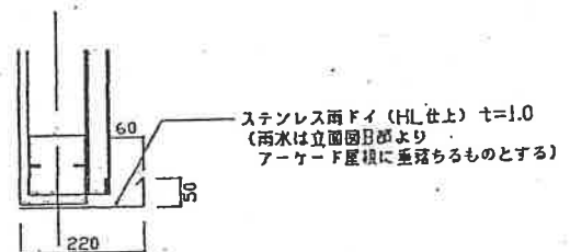
A部詳細
