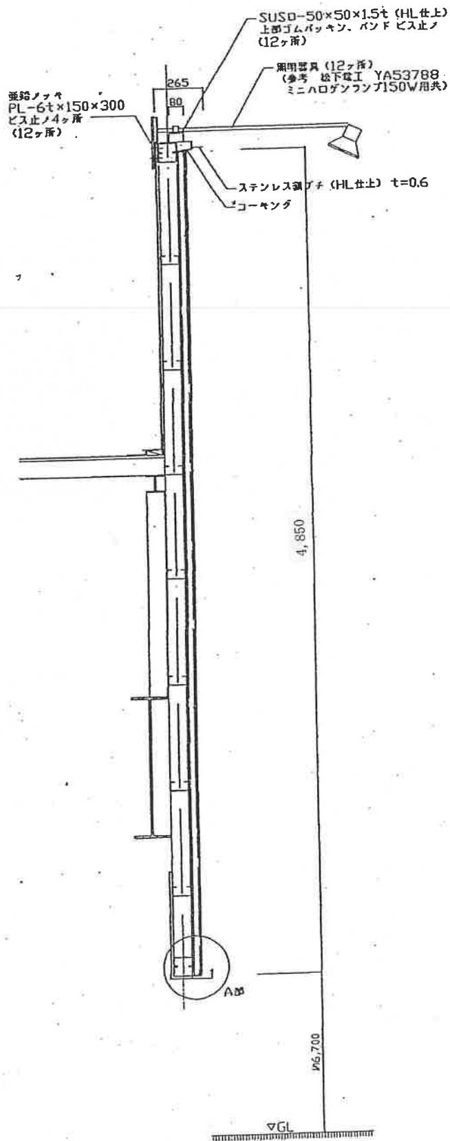
看板断面図
